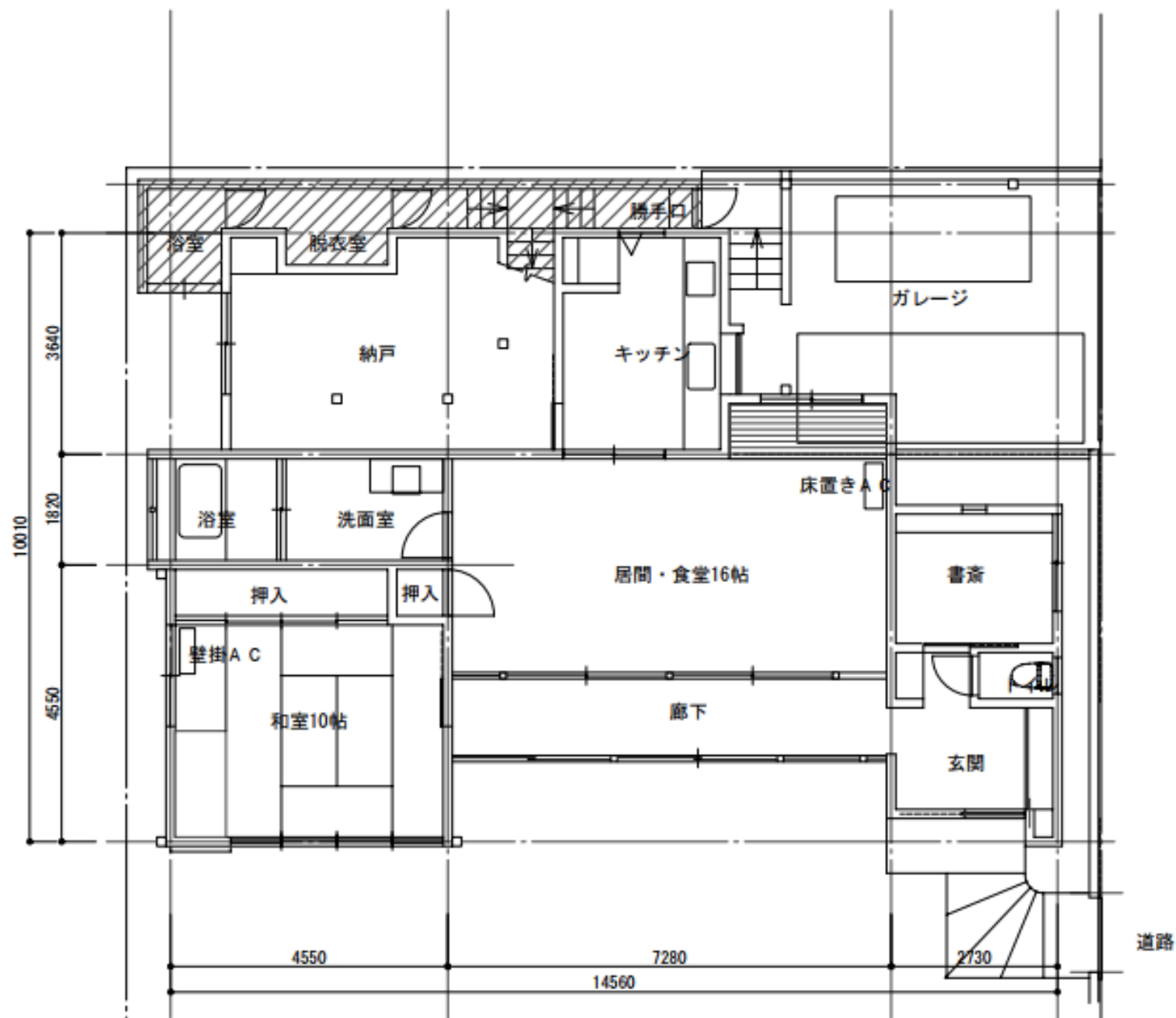
1階平面図 (106.9㎡)
