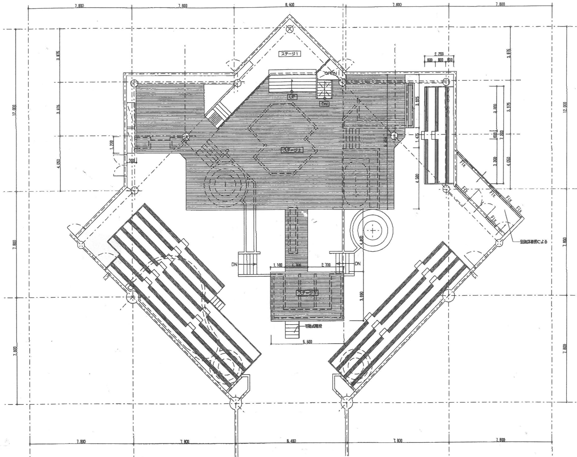
レスパール藤ヶ崎 イベントホール改修工事 完成平面図 19.03.26
