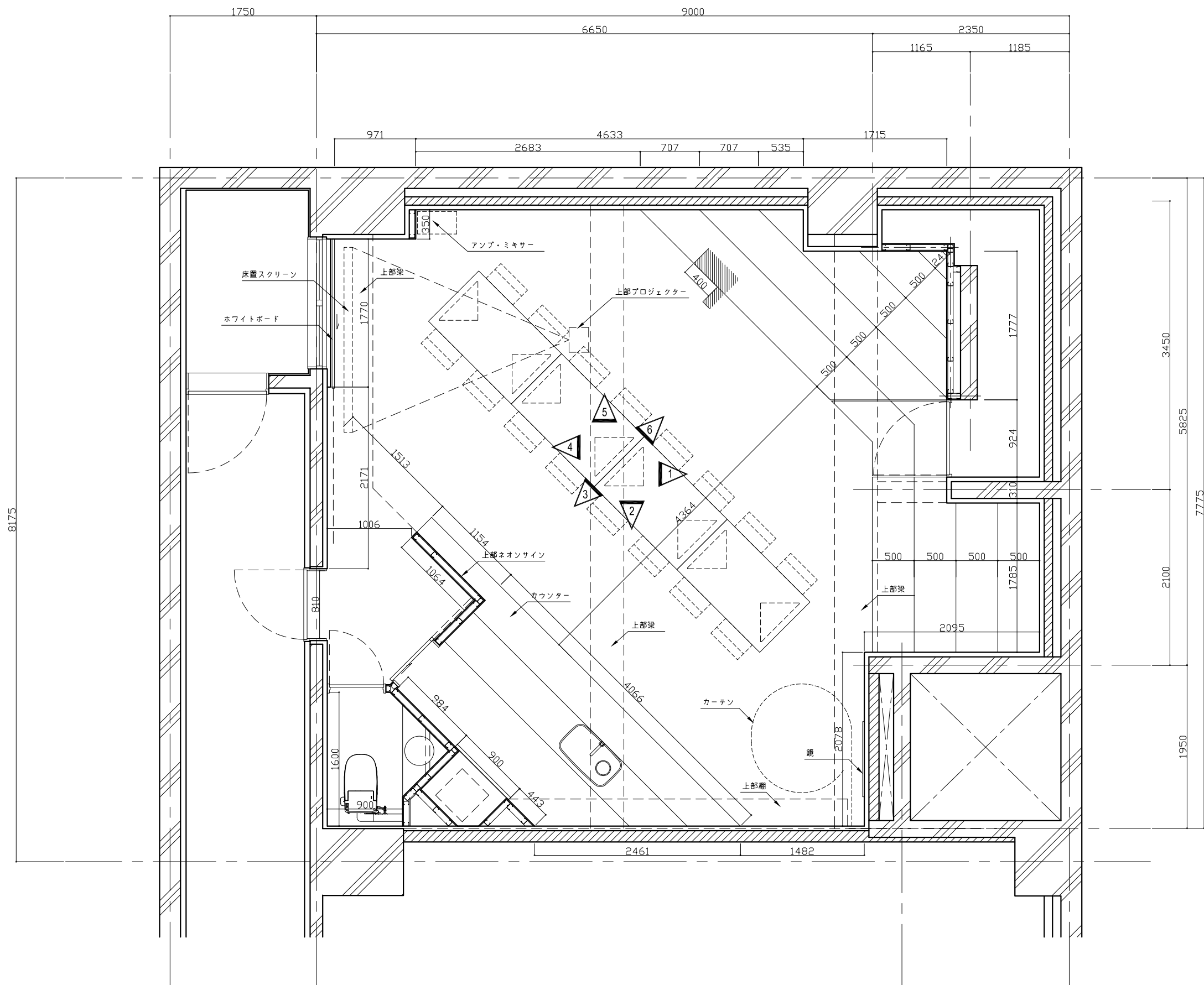
1 平面図 SCALE = 1/50(A3)
